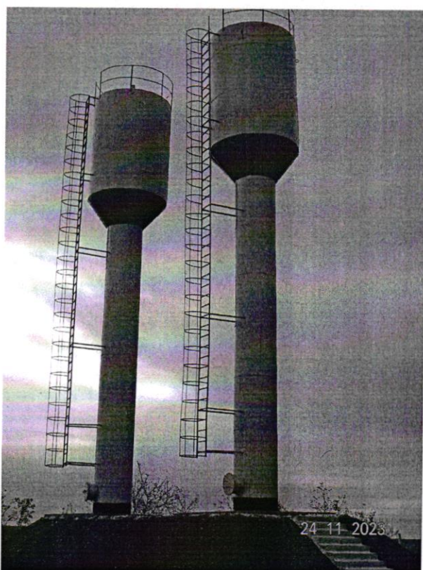
Platforma A: Volovița - 2 turnuri cu V=25m^3 și H=12m .
