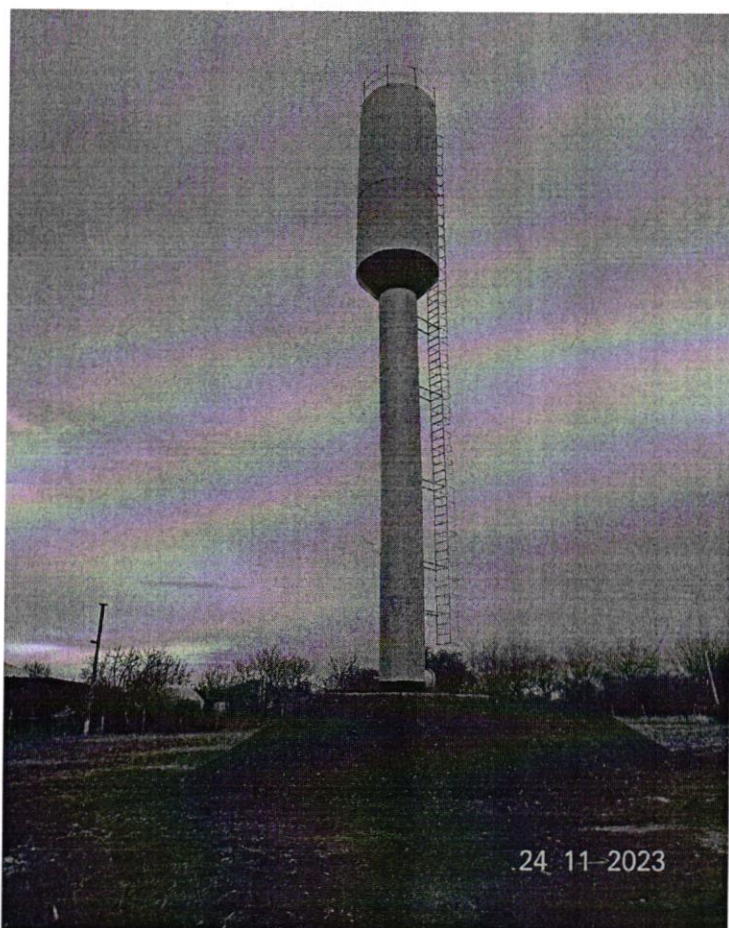
Platforma E: Racovăț - 1 turn cu V=50m^3 și H=15m .
